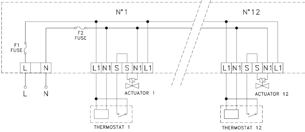
Schema electrică a distribuitorului P308/*230
