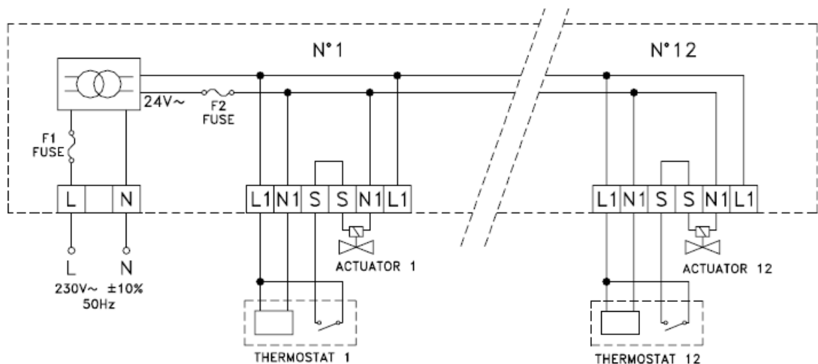
Schema electrică a distribuitorului P308*/24
